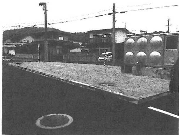
耐震貯水槽（地下埋設型）
